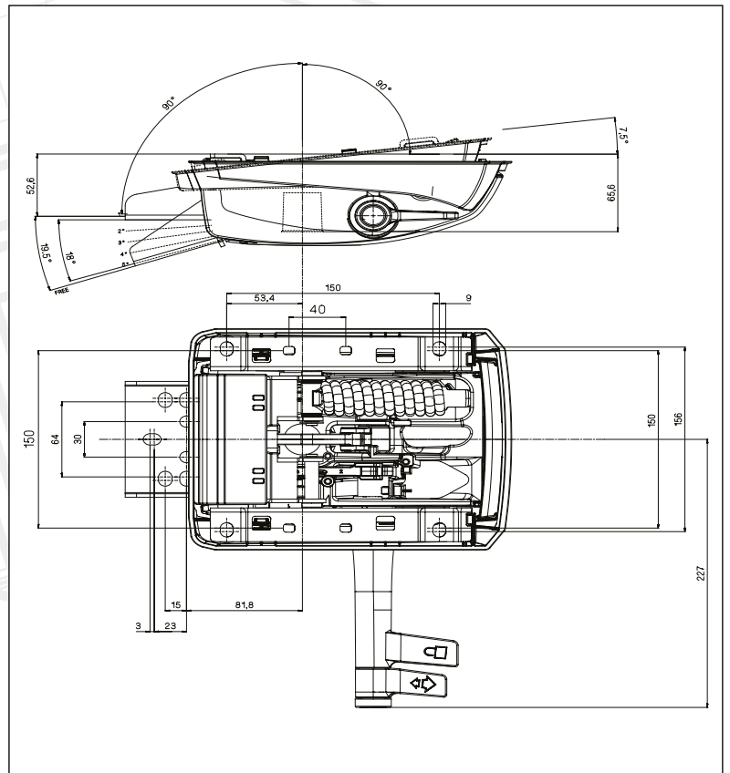
Versione senza regolazione fine della tensione Version without fine tension adjustment Modell ohne Federkraftverstellung
