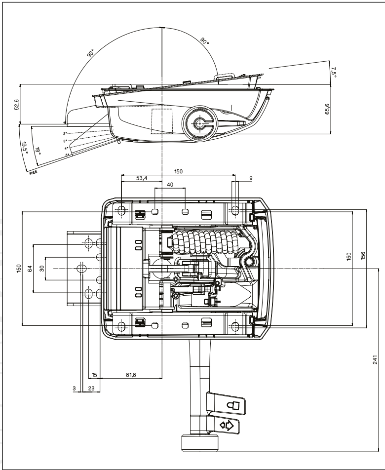
Versione con regolazione fine della tensione Version with fine tension adjustment Modell mit Federkraftverstellung
